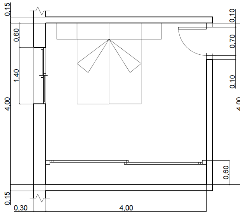
Plànol de planta del dormitori.
