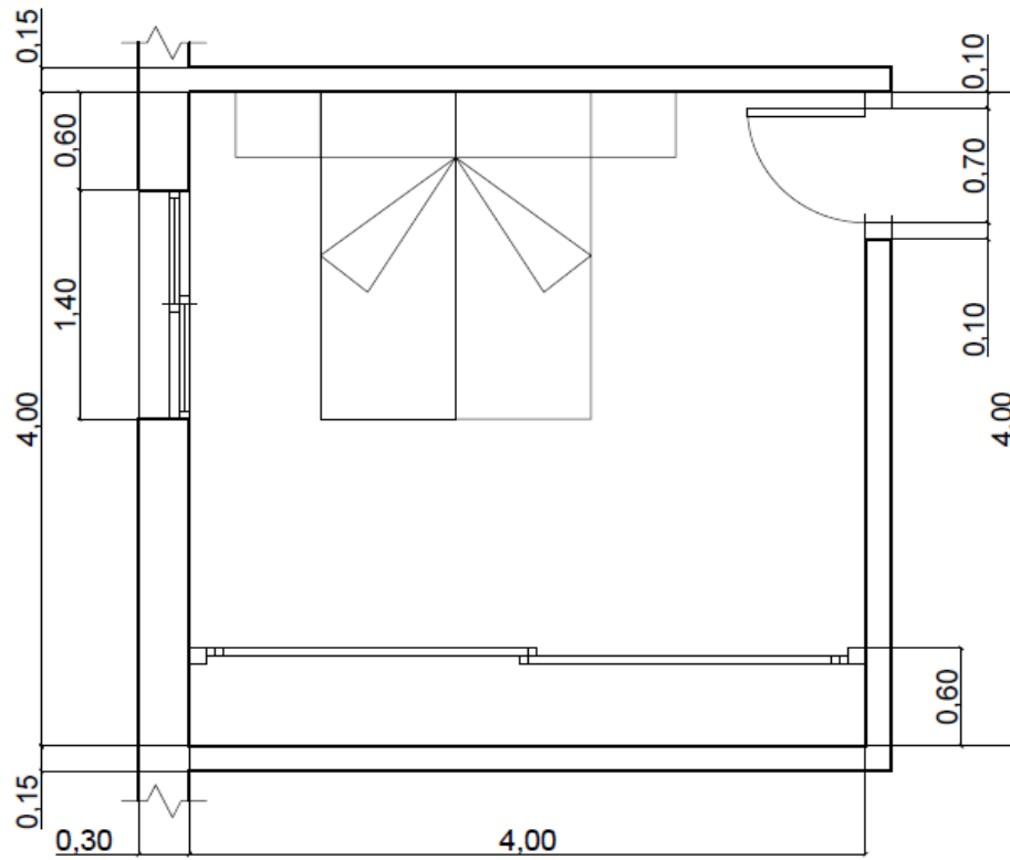
Plànol en planta a escala 1:50.
