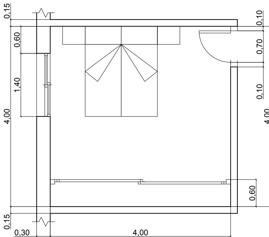
Planta del dormitori a escala 1:50
